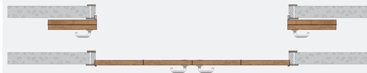
Центральное открывание для двухстворчатых дверей
