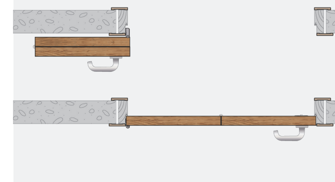
Схема складывания дверей
