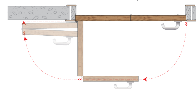
Схема складывания дверей
