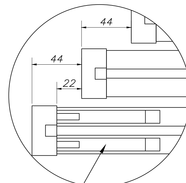
С Рекомендуемые перехлесты полотен (открытое положение)
