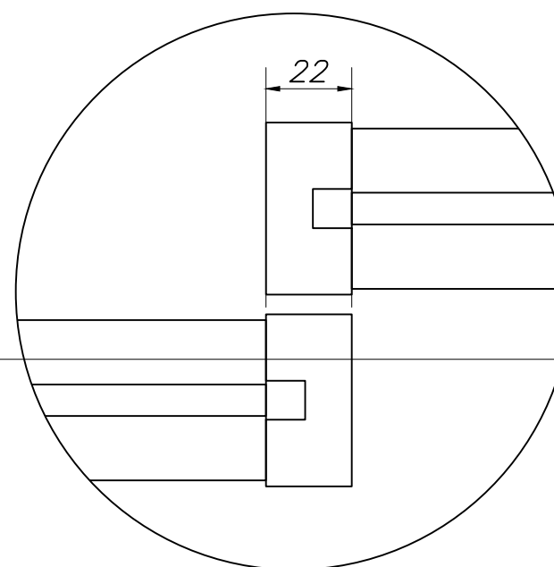
В Рекомендуемые перехлесты полотен (закрытое положение)
