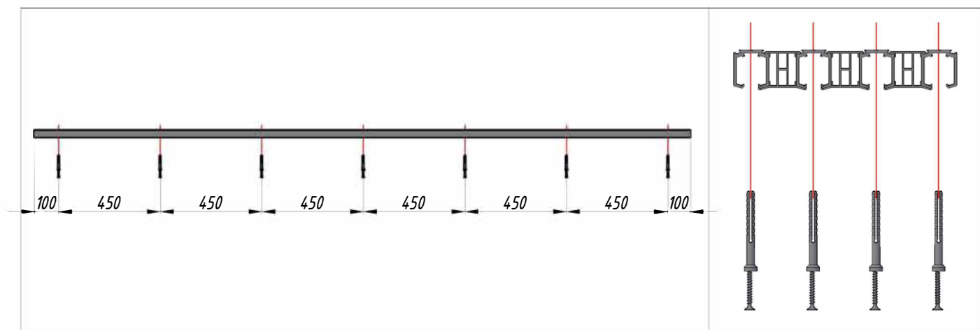
Вид спереди
