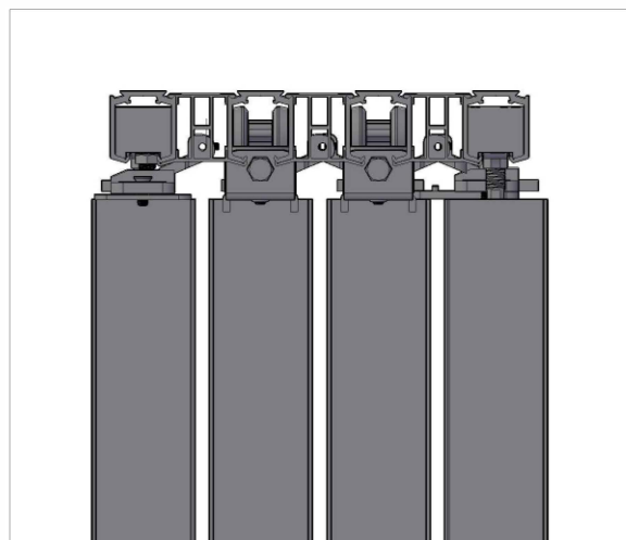
Вид справа
