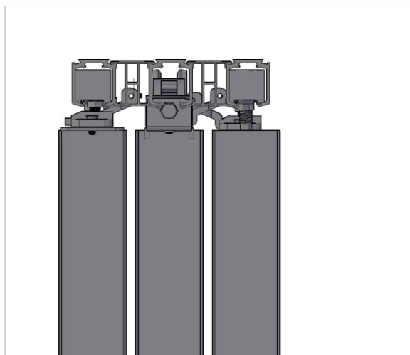
Вид справа
