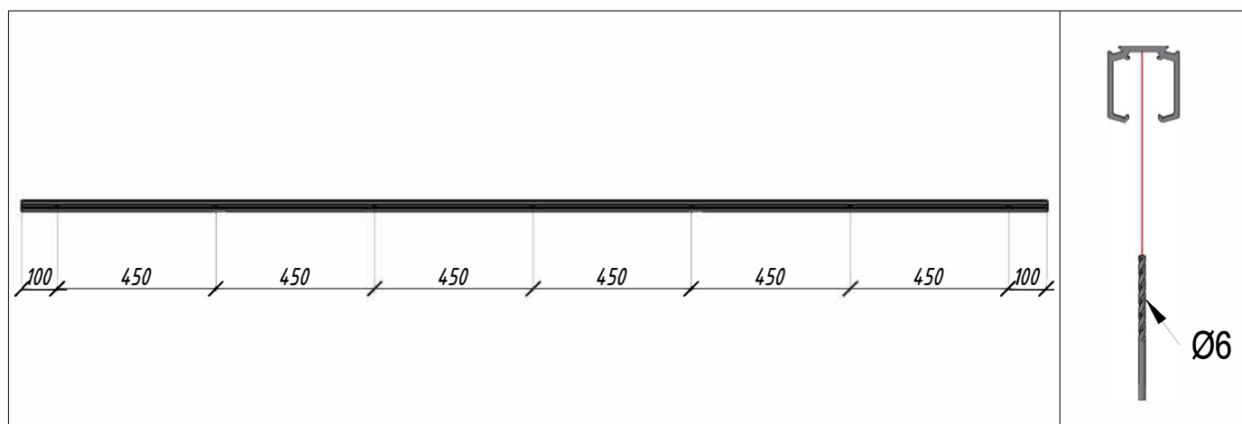
Вид снизу
